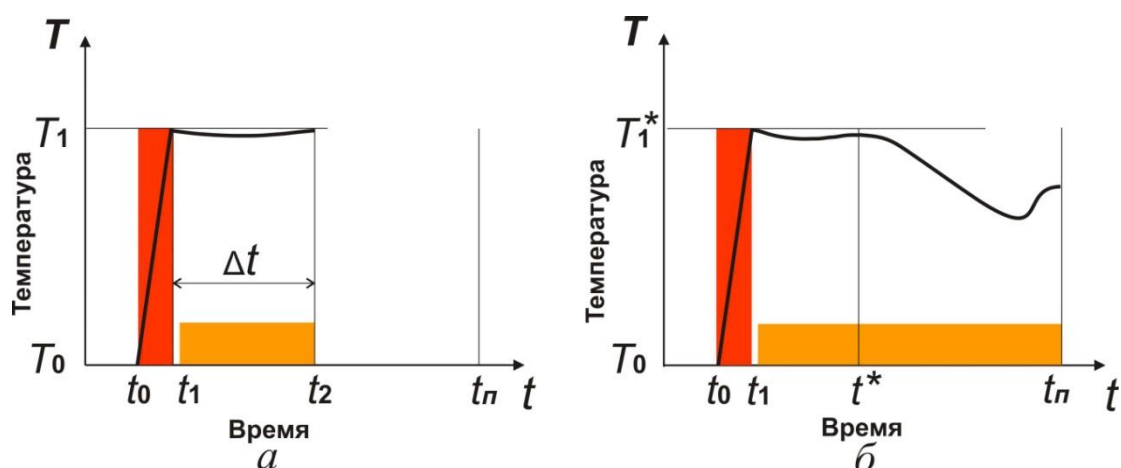
Рис. 5. Характерные траектории нагрева зонда в жидкости при условиях t_2 < t_{\Pi} (рис. а) и t_2 > t_{\Pi} > t^* (рис. б). Здесь t_1 и t_2 – моменты баланса моста, между которыми осуществляется отсчет времени; t_{\Pi} – полная продолжительность нагрева. Длительности участков нагрева ( t_0 \div t_1 ) и измерения ( \Delta t ) составляют 10^{-5} с и 10^{-3} с, соответственно. Тенью условно показано соотношение мощностей нагрева на первом и втором участке.
