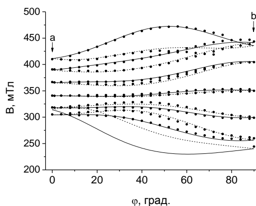
Рисунок 13 - Ориентационное поведение резонансных положений переходов двух триклинных центров \text{Gd}^{3+} в плоскости ab . Точки – эксперимент, кривые – расчет с параметрами таблицы 3
