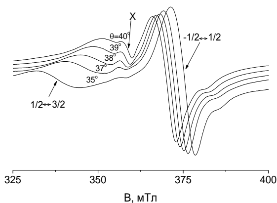
Рисунок 7 - Зависимость от полярного угла \theta в плоскости zy вида ЭПР спектра в районе пересечения переходов \pm 1/2 \leftrightarrow \pm 3/2 при 300К. Сигналы переходов -1/2 \leftrightarrow -3/2 не наблюдаемы из-за доминирующих по интенсивности сигналов -1/2 \leftrightarrow +1/2
