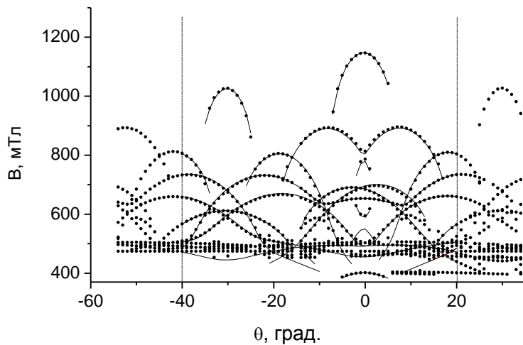
Рисунок 4 - Полярная угловая зависимость положений переходов центров \text{Gd}^{3+}\text{-F}^- в германате свинца при \mathbf{B} \perp \mathbf{C}_3 (в плоскости \mathbf{zx} ). Точки – эксперимент, кривые – расчет с константами таблицы 4.1 в диапазоне 60^\circ для трех центров, отличающихся поворотом на 120^\circ вокруг \mathbf{C}_3 . Низкополевая область спектра не приводится, поскольку она занята интенсивными сигналами одиночного центра \text{Gd}^{3+} и переходами центров \text{Gd}^{3+}\text{-Cl}_i^- и \text{Gd}^{3+}\text{-O}_i^{2-}
