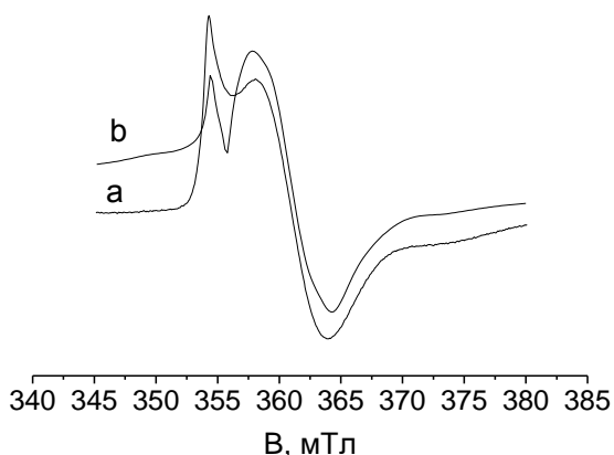
Рисунок 10 - Форма ЭПР спектра в районе переходов -1/2 \leftrightarrow +1/2 (300К, \theta = 10^\circ ). а – эксперимент, б – симуляция с использованием выражения (6)
