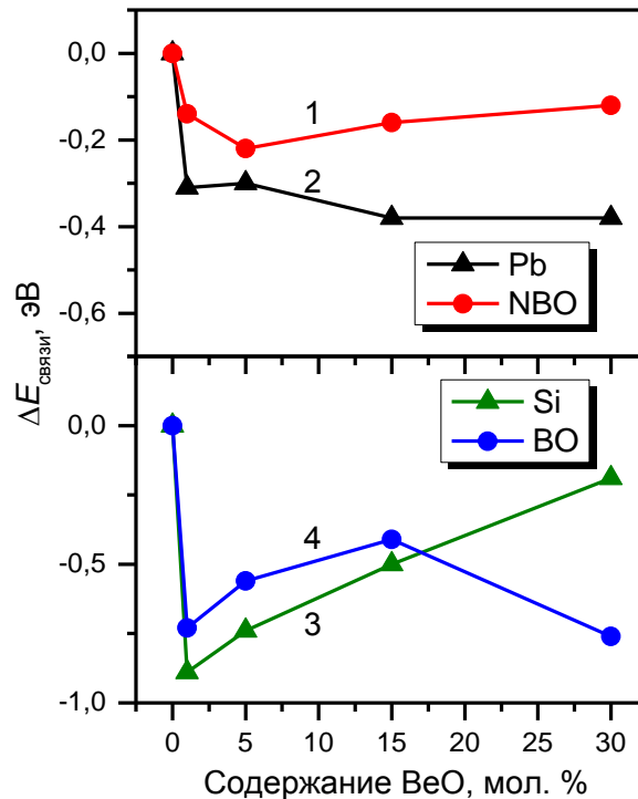
Рис. 7. Концентрационные зависимости разностей энергий связи РФЭС линий исходного стекла 50PbO-50SiO 2 и стекло BeO-PbO-SiO 2 : (1) – 1 нестикового кислорода, (2) – 4f свинца, (3) – 2p кремния и (4) – 1s мостикового кислорода
