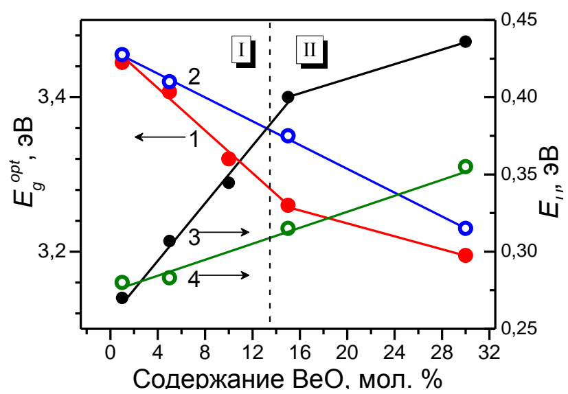
Рис. 10 Влияние содержания \text{BeO} на энергетические характеристики: (1),(2) – оптическая ширина запрещенной зоны E_g^{\text{opt}} по Тауцу; (3),(4) – энергия Урбаха E_U . (1),(3) – после воздействия быстрыми нейтронами; (2),(4) – до облучения
