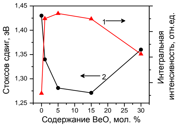
Рис. 8. Концентрационные зависимости интенсивности ФЛ (1) и стоксова сдвига ФЛ (2).
