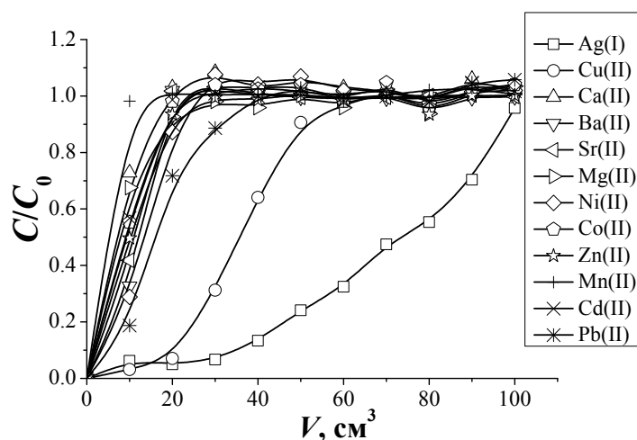
Рисунок 6 – Динамические выходные кривые сорбции ионов металлов СЭХ 1.0. Одновременное присутствие ионов металлов в растворе. C_{исх}(Me) = (1 \div 2) \cdot 10^{-4} моль/дм 3 . Аммиачно-ацетатный буферный раствор, pH=6.5. g_{сорб} = 0.1000 г. Скорость пропускания раствора 1 см 3 /мин
