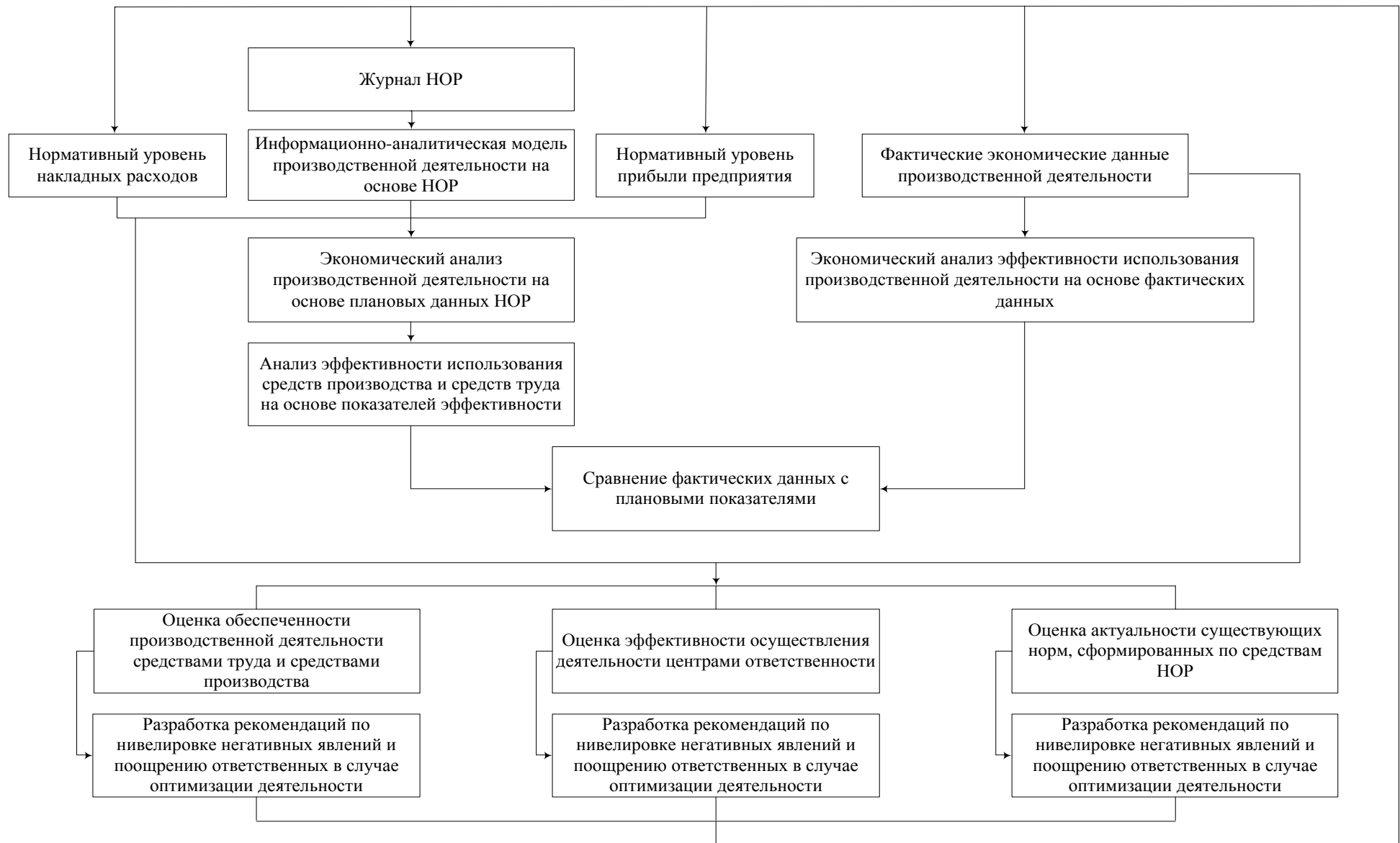
Рисунок 4 – Порядок реализации аналитической экономико-математической модели
