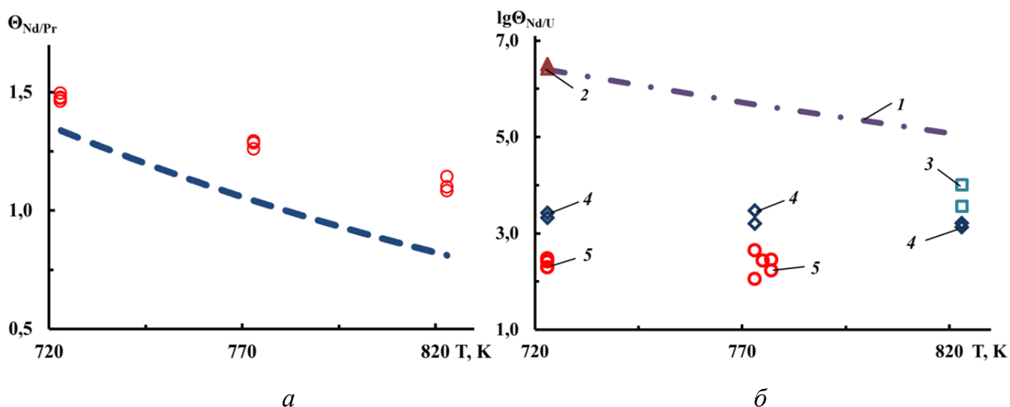
Рисунок 2 – Результаты верификации КР пар « Nd/Pr » (а) , « Nd/U » (б) в системе «эвтектический сплав Ga-Sn – солевой хлоридный расплав»: пунктирные линии – расчетные значения КР, точки – экспериментальные значения КР
