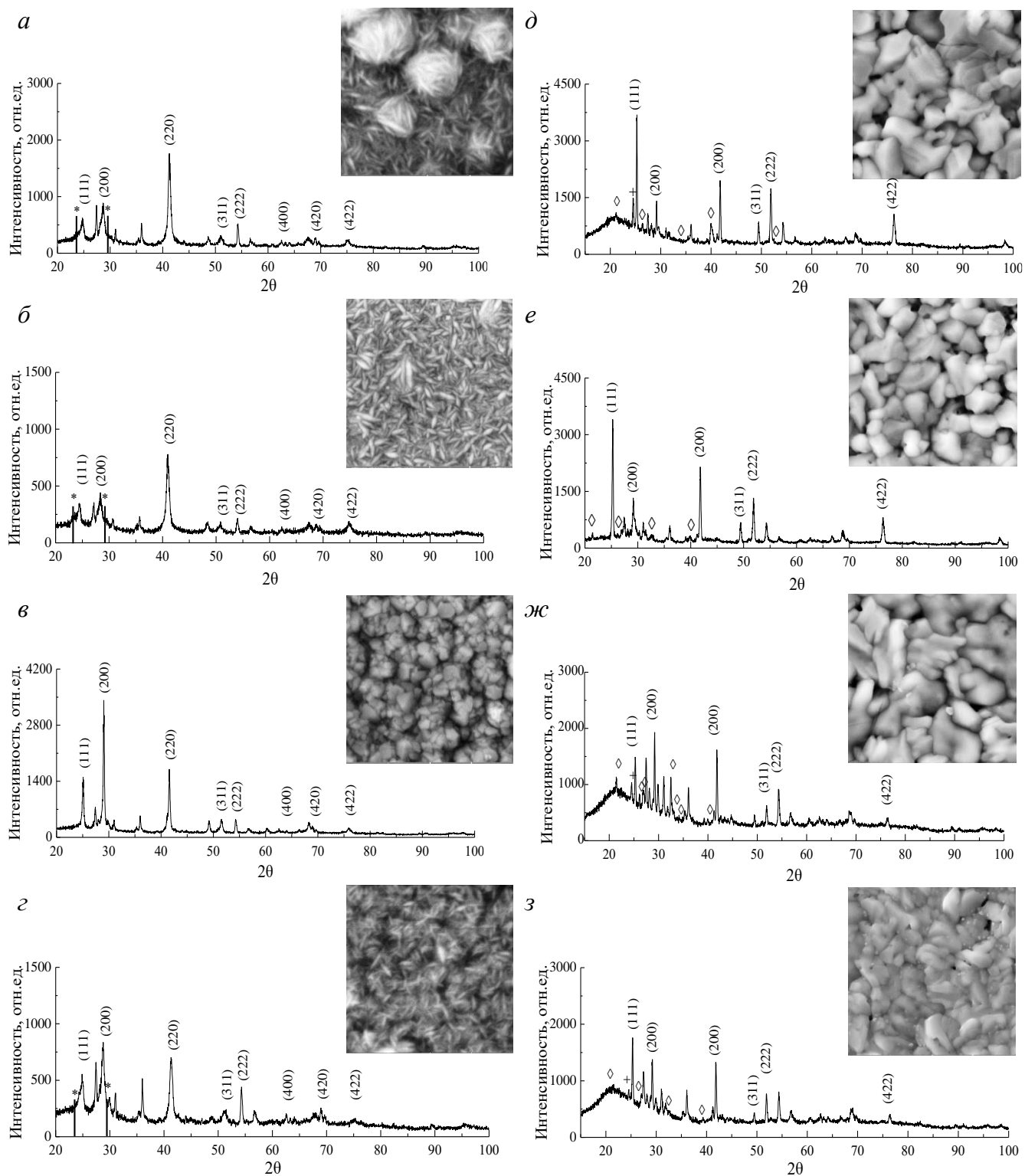
Рис. 4. Рентгенограммы и микроизображения свежесаженных ( а, б, в, г ) и термообработанных ( д, е, ж, з ) пленок PbSe(I), синтезированных в присутствии антиоксидантов: Na 2 SO 3 ( а, д ), Na 2 SO 3 + C 6 H 8 O 6 ( б, е ), C 6 H 8 O 6 ( в, ж ) и SnCl 2 ( г, з ).
