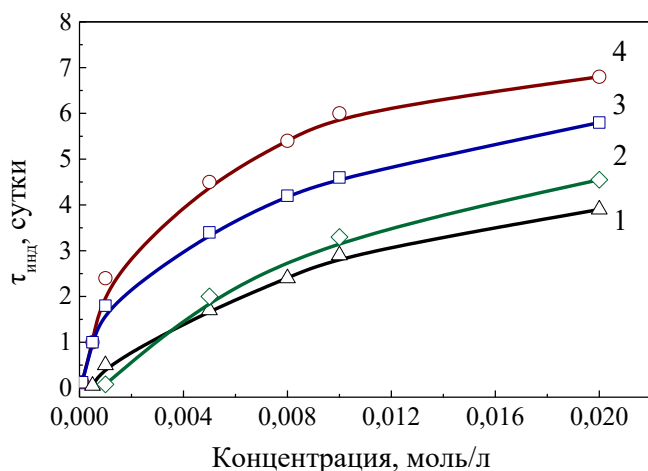
Рис. 2. Зависимость индукционного периода окисления водного раствора селеномочевины кислородом воздуха от концентрации антиоксиданта \text{Na}_2\text{SO}_3 (1); \text{SnCl}_2 (2); \text{C}_6\text{H}_8\text{O}_6 (3); смеси \text{Na}_2\text{SO}_3 + \text{C}_6\text{H}_8\text{O}_6 (4).
