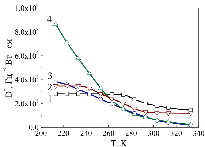
Рис. 7. Температурная зависимость обнаружительной способности фоточувствительных элементов на основе PbSe(I), полученных гидрохимическим осаждением с использованием Na 2 SO 3 (1), Na 2 SO 3 + C 6 H 8 O 6 (2), C 6 H 8 O 6 (3) и SnCl 2 (4). Температура отжига 653 К. Размеры чувствительных элементов 2 \times 2 мм
